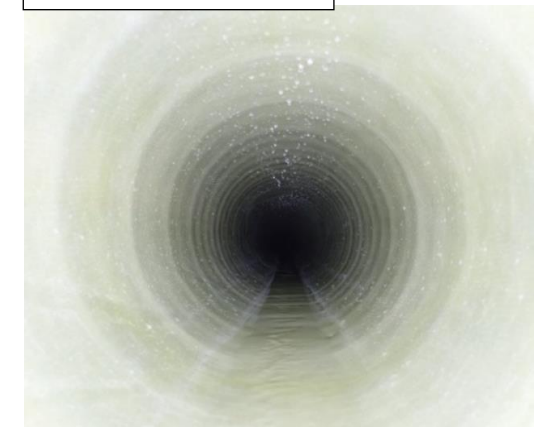
管更生した管（施工後）
